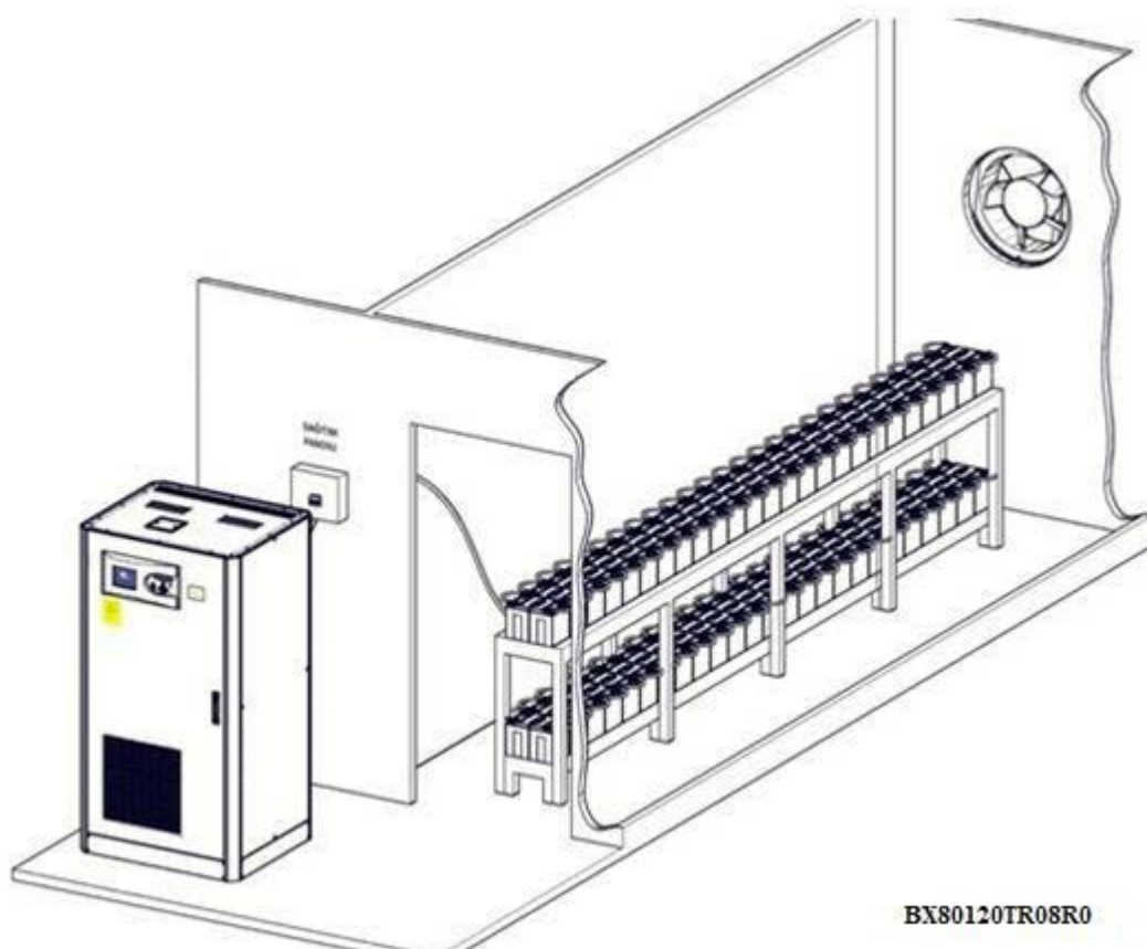
Размещение внешних АКБ на стеллажах
