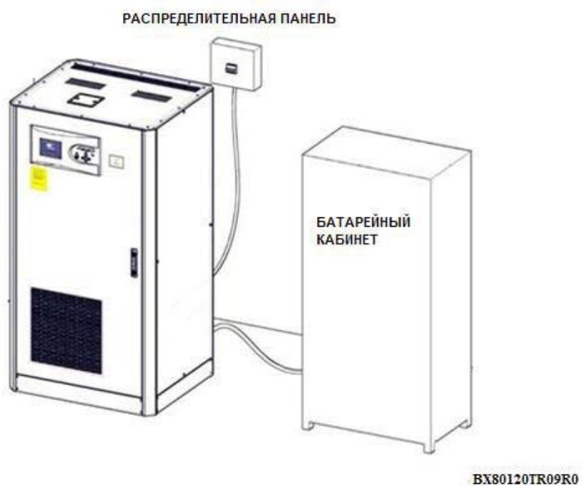
Размещение внешних АКБ в кабинете
